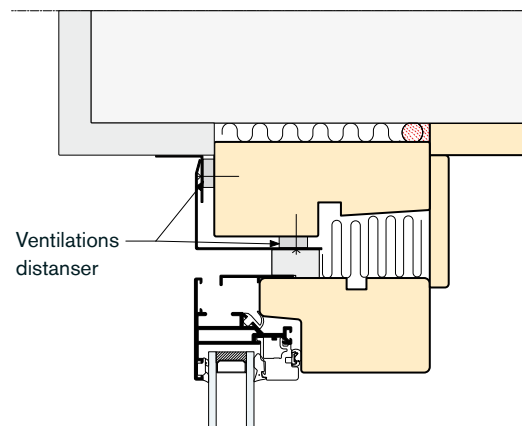
VELFAC • 00i monterat i befintligt inåtgående fönster
