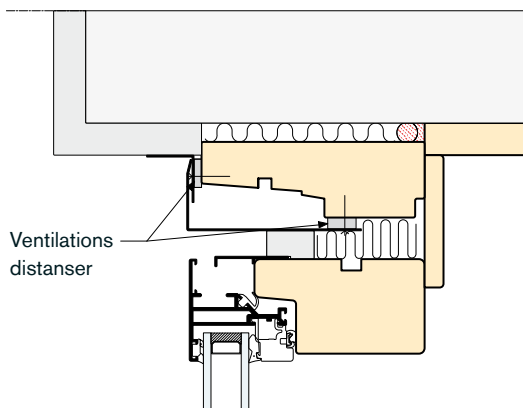
VELFAC • 00i monterat i befintligt utåtgående fönster
