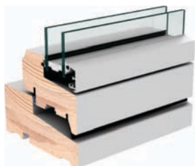
VELFAC Ribo træ, 2-lags
